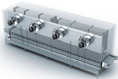
+ Congelador Impingement
